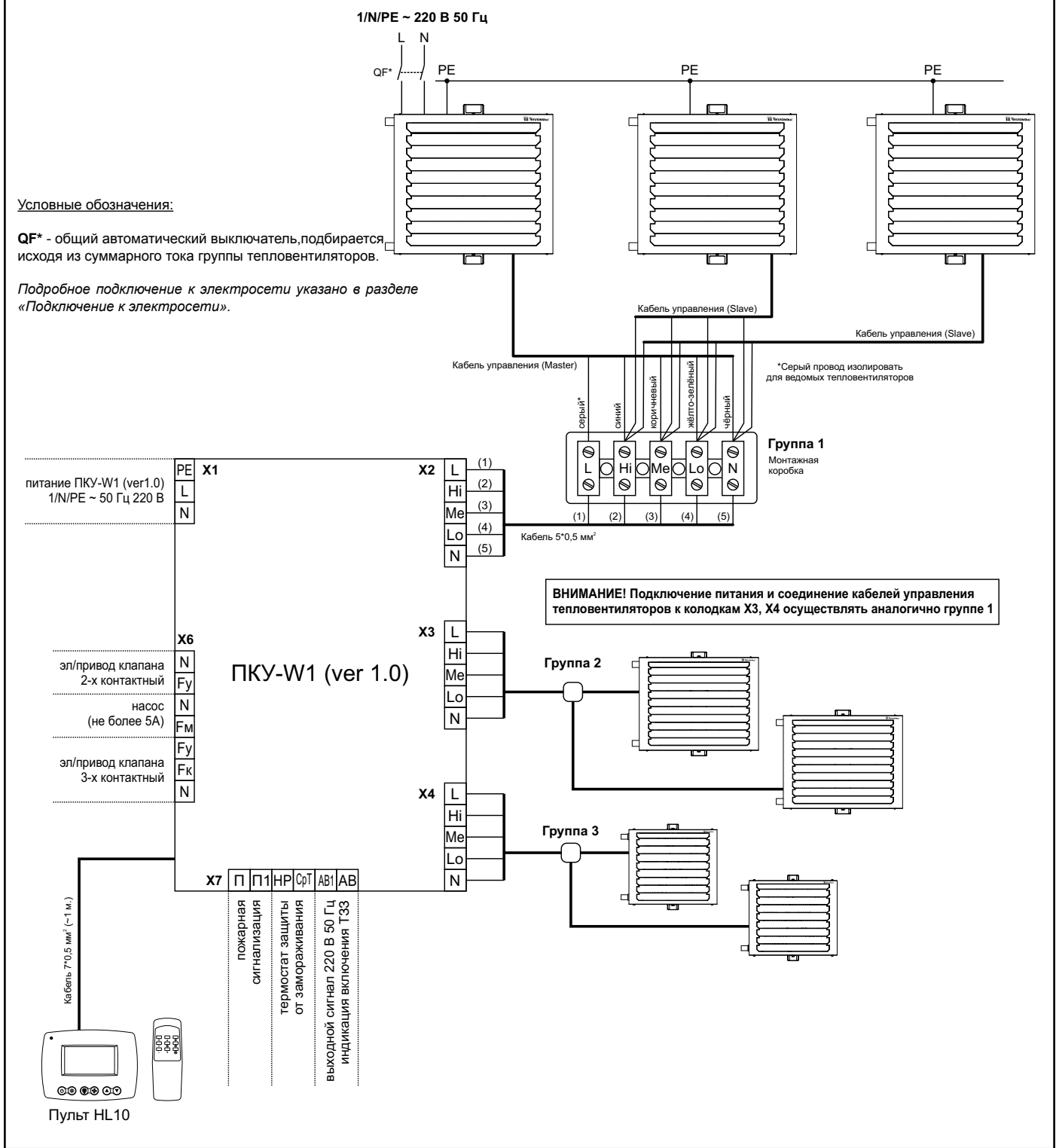
Схема подключения групп тепловентиляторов к ПКУ-W1 (ver1.0)
